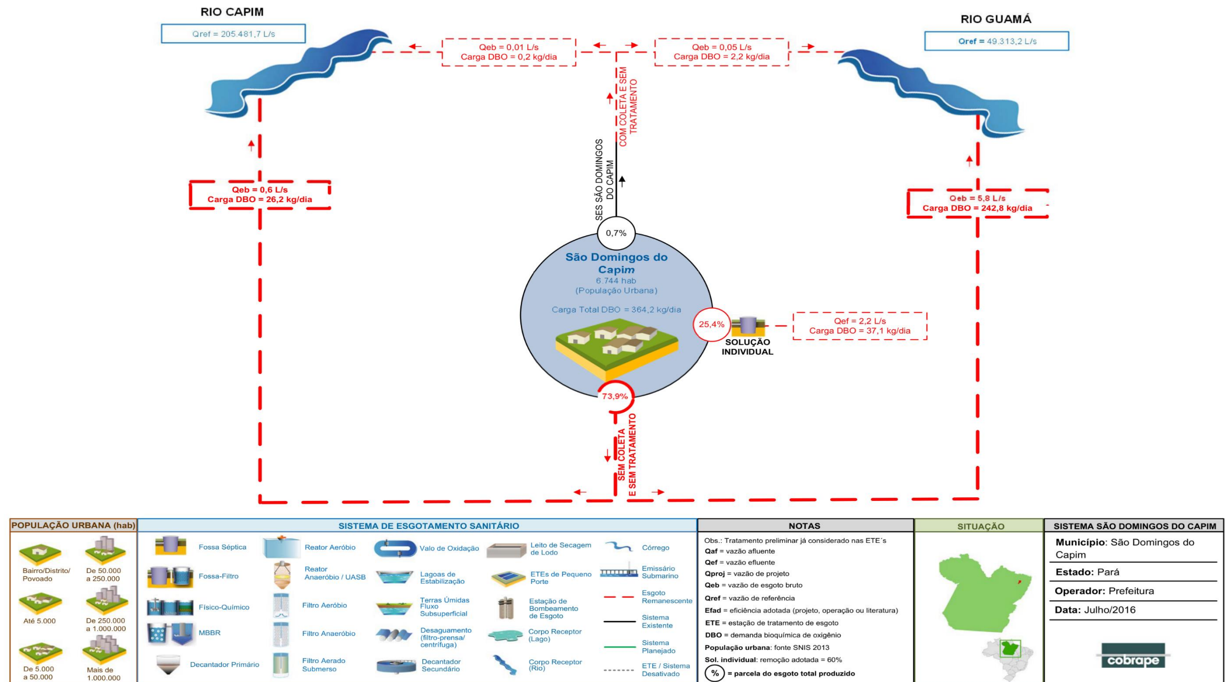
Figura 2. Diagrama do Sistema de Esgotamento Sanitário (SES). Fonte: Retirado de ANA, 2023.
