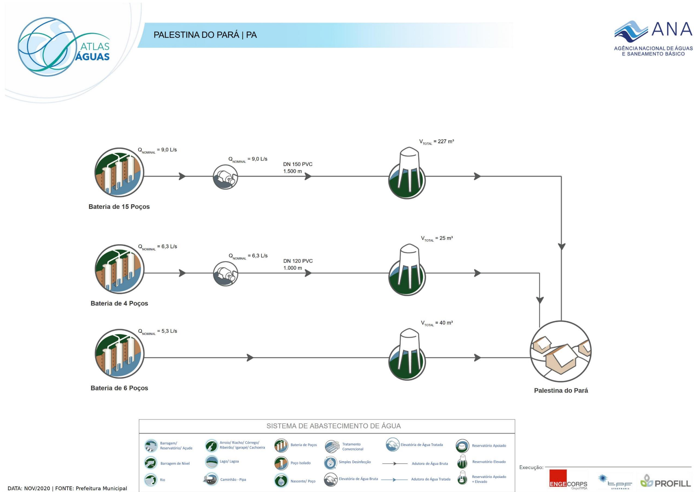
Figura 1. Diagrama do Sistema de Abastecimento de Água (SAA).
