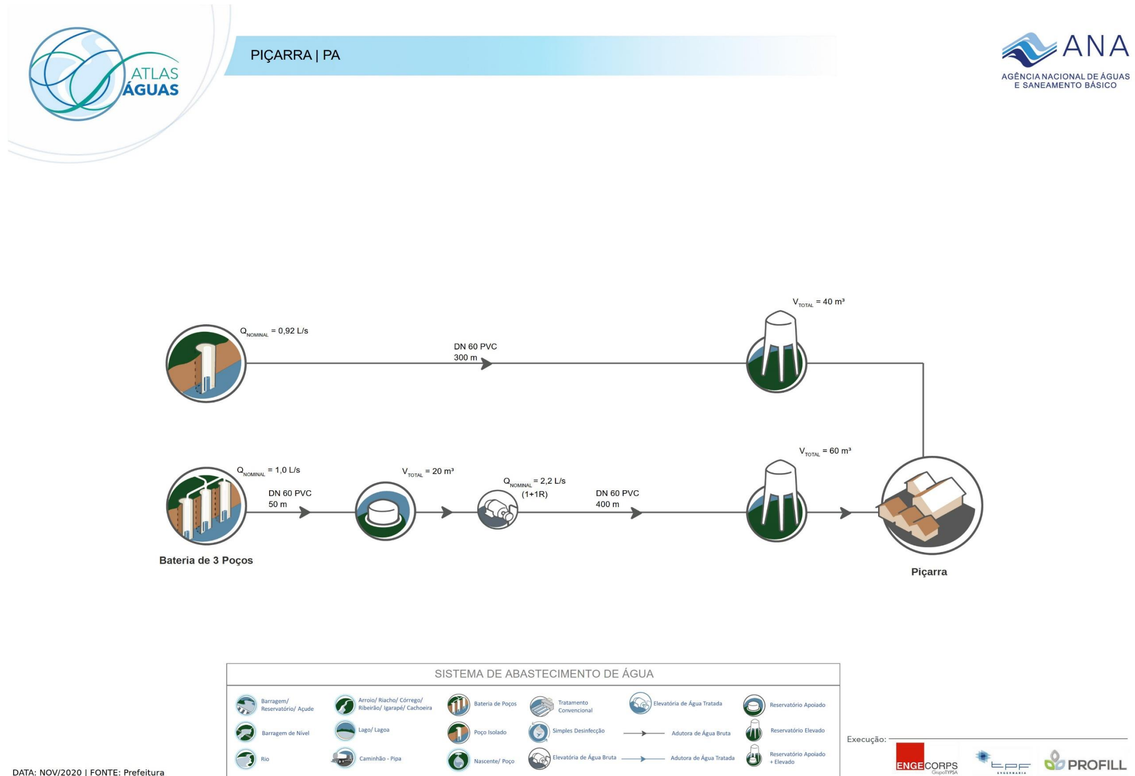
Figura 1. Diagrama do Sistema de Abastecimento de Água (SAA). Fonte: Retirado de ANA, 2023.
